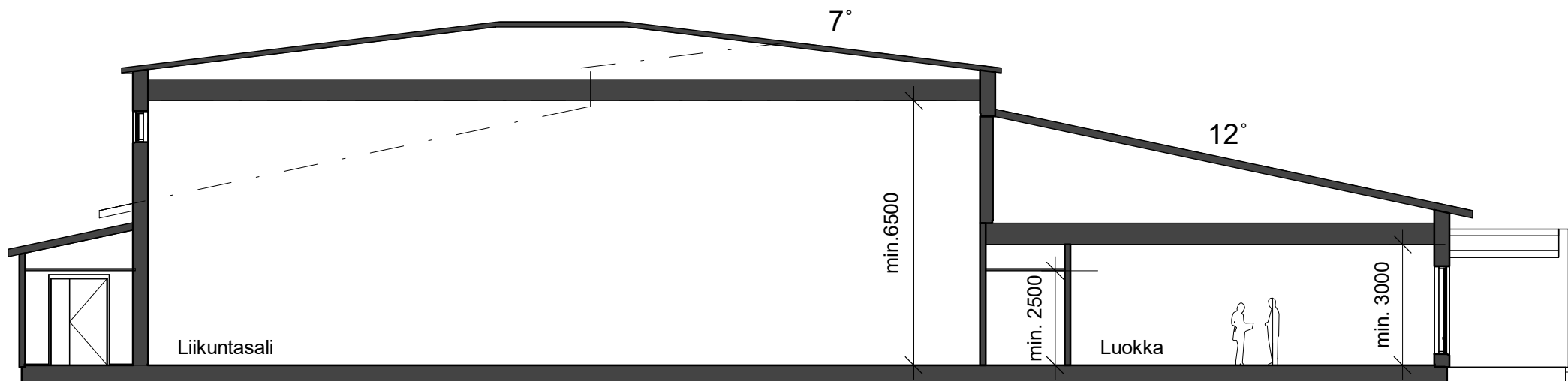
A-A Leikkaus 1 : 150
